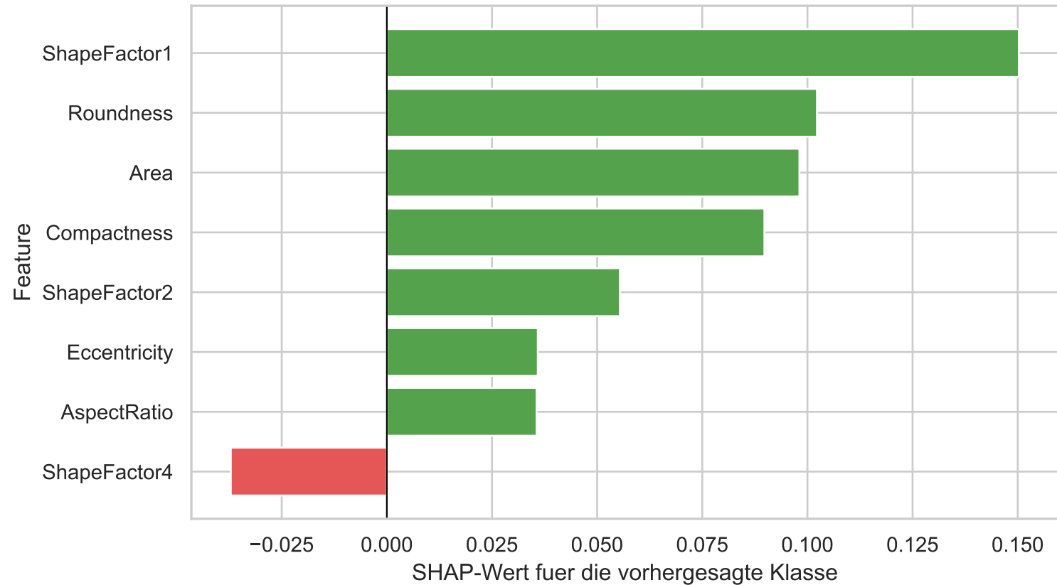
Lokale SHAP-Fehlklassifikation: DERMASON als SIRA
